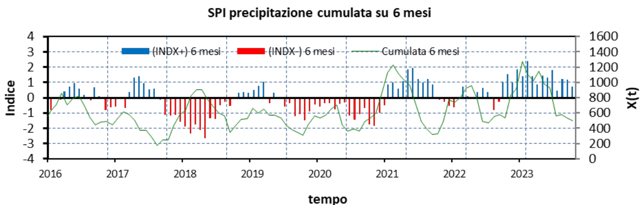
Figura 29. Pluviometro di Caposele - SPI su 6 mesi
