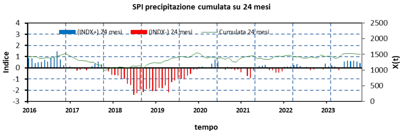
Figura 48. Pluviometro Tarsia - SPI su 24 mesi
