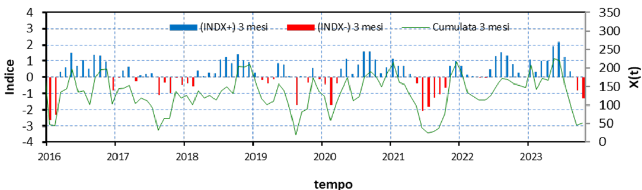
Figura 71. Pluviometro Foggia Osservatorio - SPI su 3 mesi
