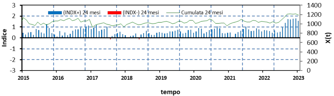
Figura 74. Pluviometro Foggia Osservatorio - SPI su 24 mesi
