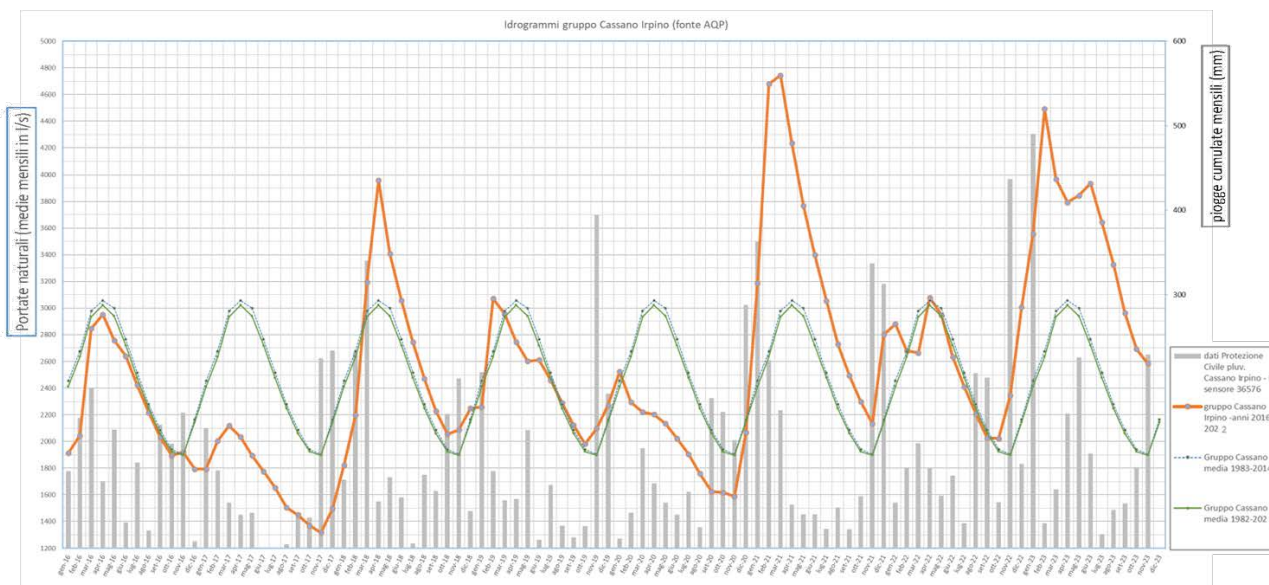
Figura 18. Andamento delle portate naturali in relazione alle piogge cumulate per il Gruppo Sorgivo Cassano Irpino
